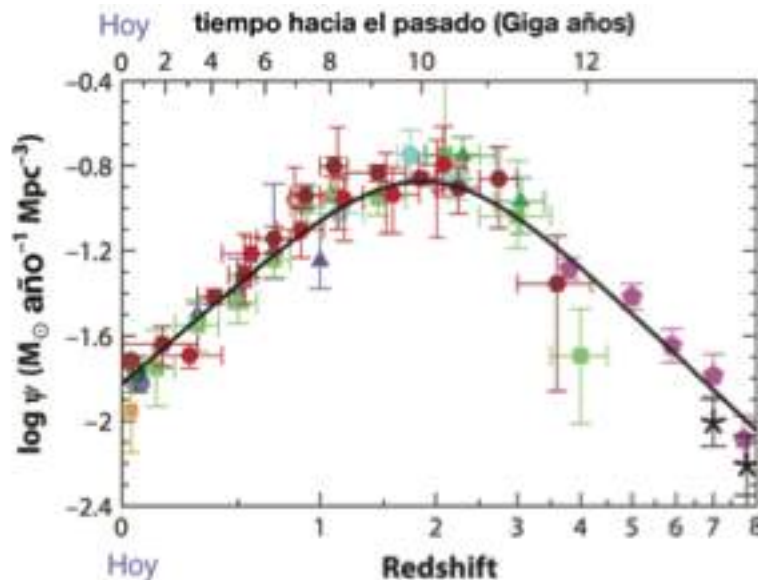
Evolución del ritmo de formación estelar en el universo (Madau & Dickinson 2014).
