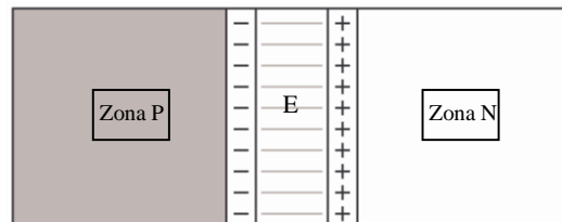
Figura 1. Creación de un campo eléctrico en la junta.
