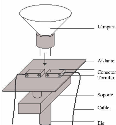
Figura 5. Esquema del portalámpara.
