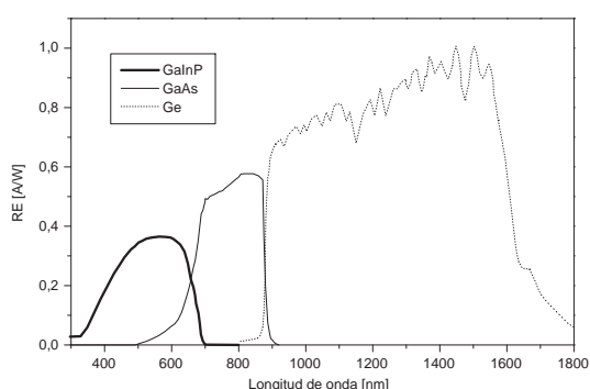
Figura 9. RE de una celda triple juntura GaInP-GaAs-Ge obtenida de la literatura [6] . La tabla fue recuperada con técnicas de tratamiento grafico.
